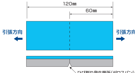
JHS 417-1999 日本道路公園規格 「コンクリート塗装材の品質規格試験方法 4.7 ひび割れ追従性試験」準拠
