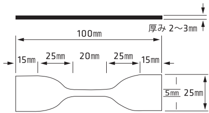
JIS K 6251 引張試験片の形状： ダンベル3号形
