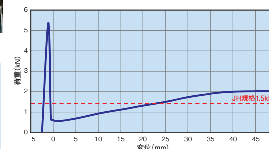
押抜き試験
